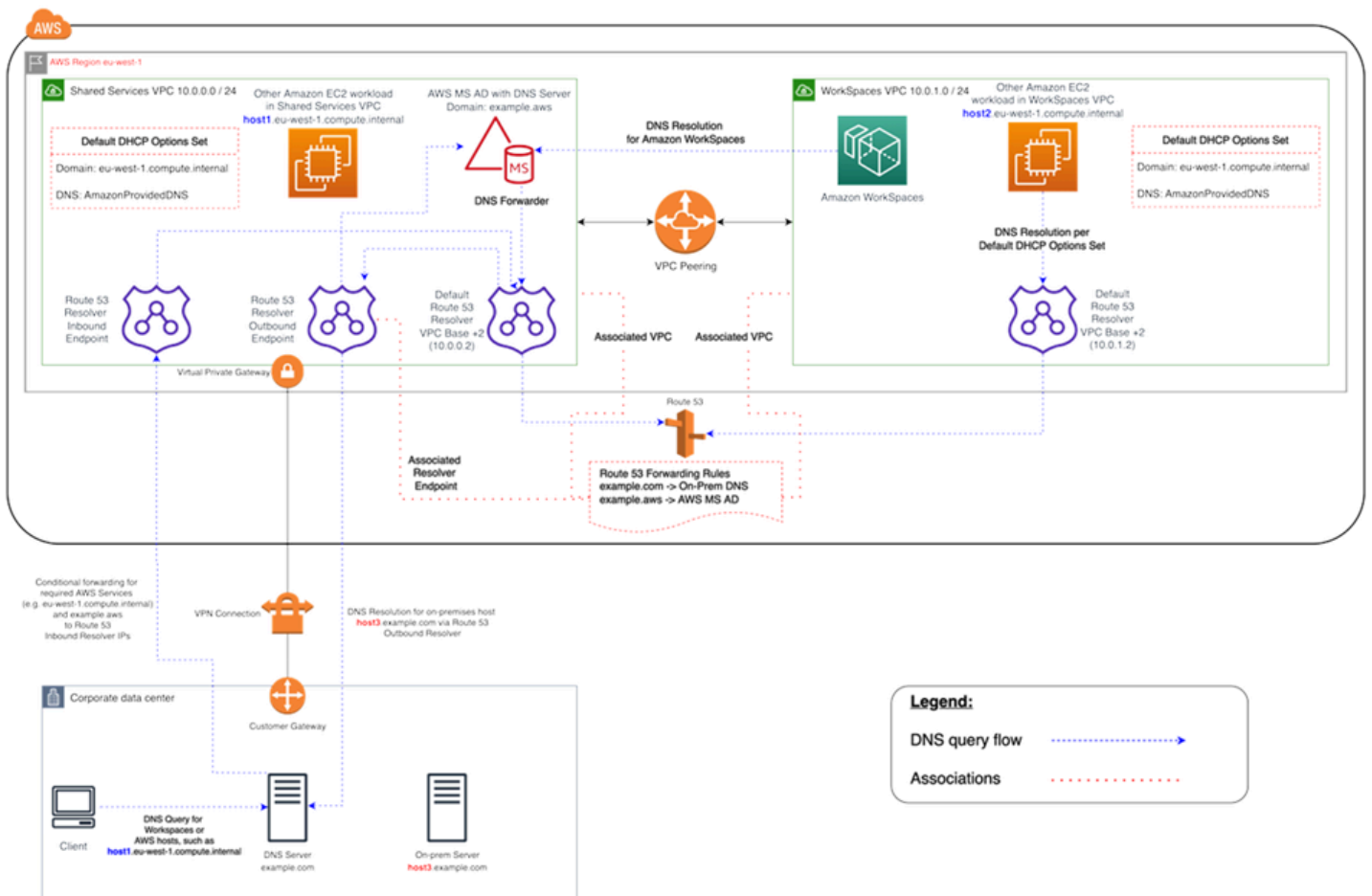
Figura 2: esempio di risoluzione WorkSpaces DNS con endpoint Route 53
