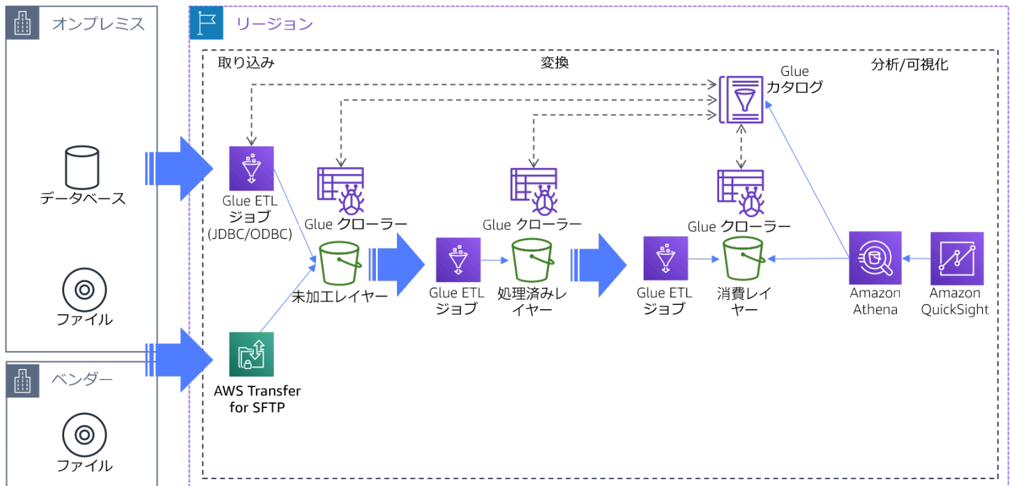
図 2: 金融サービス業界のデータレイクのリファレンスアーキテクチャ
