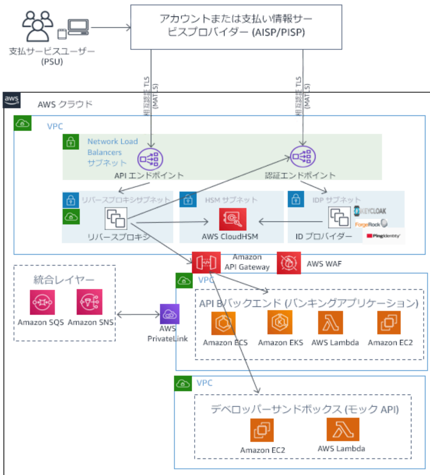
図 5: オープンバンキングのリファレンスアーキテクチャ
