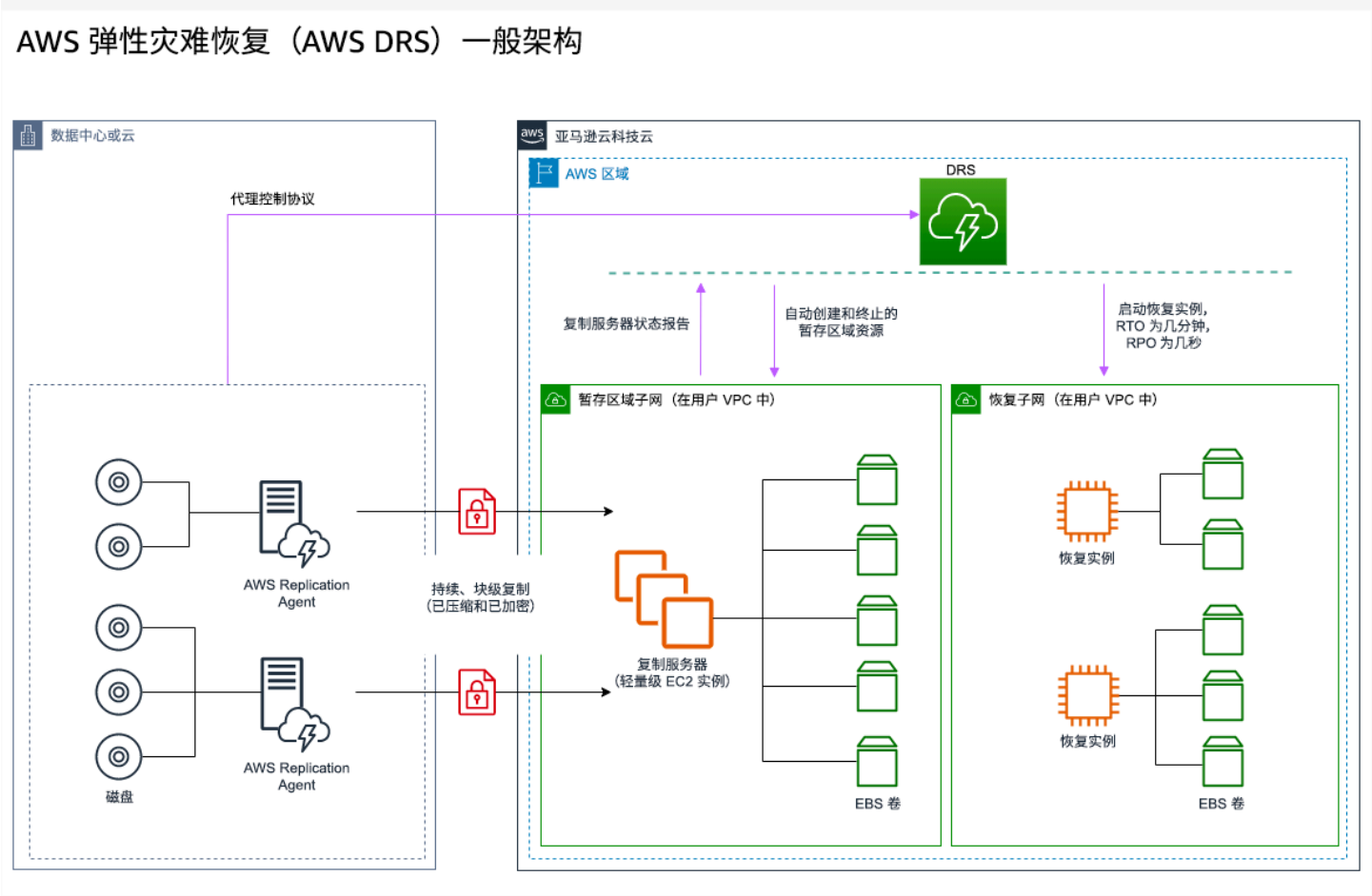
图 23 : AWS Elastic Disaster Recovery 架构
